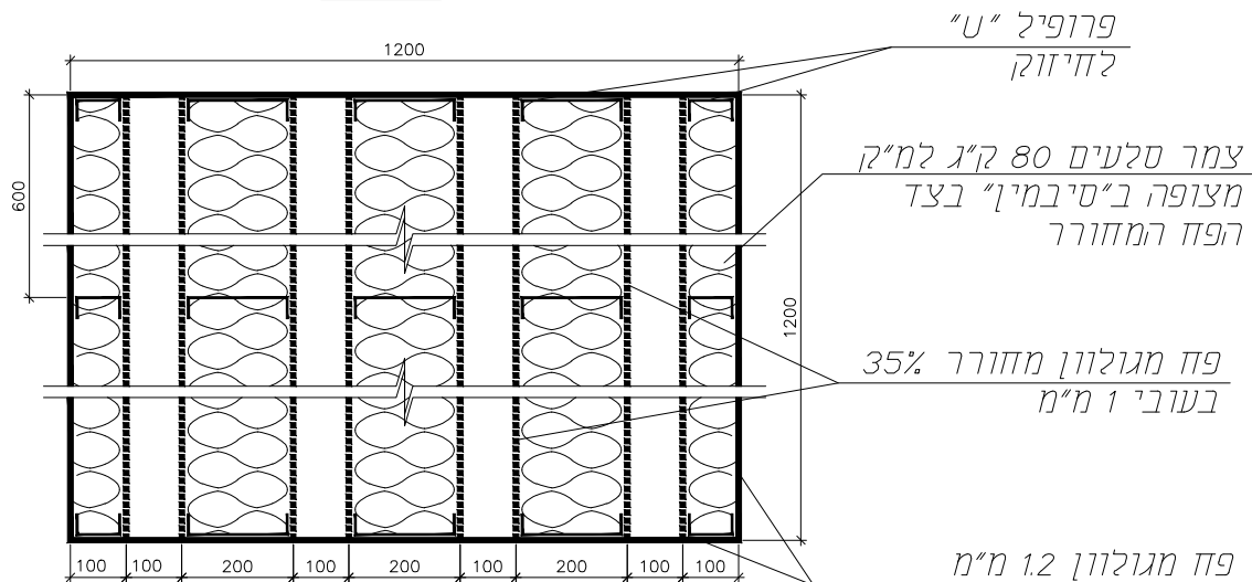
חותך 1-1
