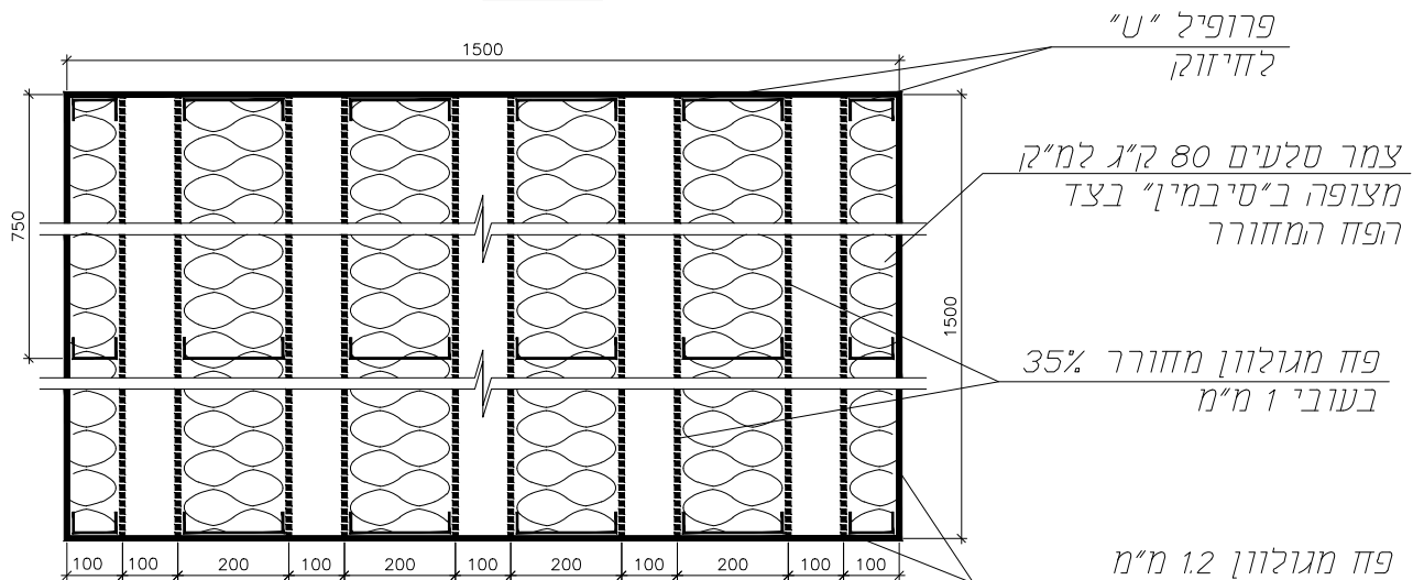
חתך 1-1
