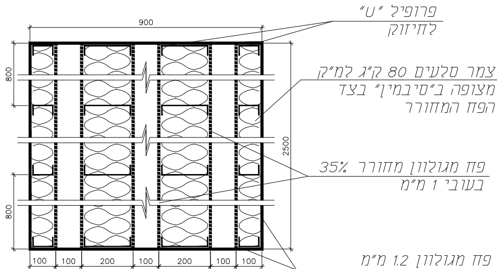
חתך 1-1
