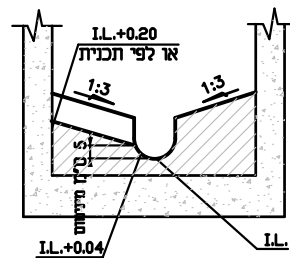
חתך ב-ב
