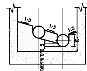
חתך א-א
