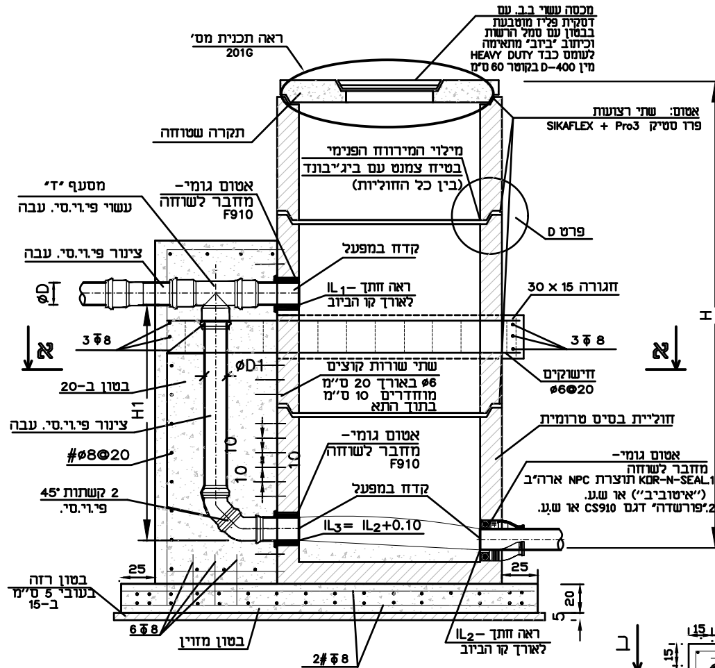
חתך ב-ב
