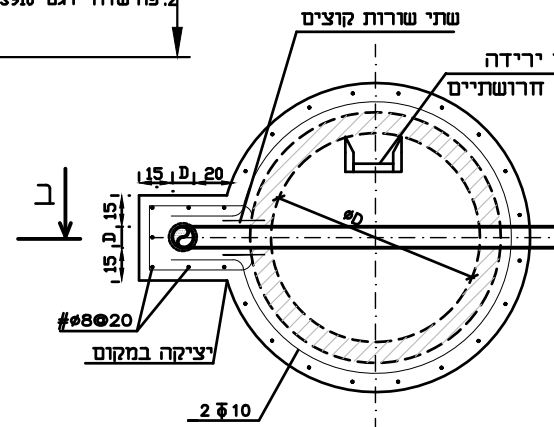
חתך א-א
